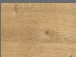
dub sukatý (PD)
